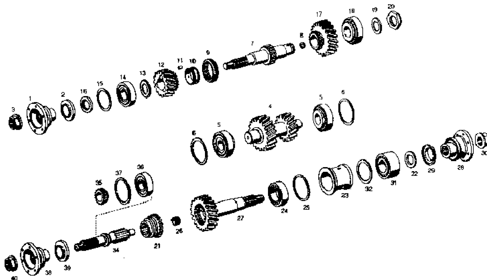
GEAR SHAFTS AND GEARS (AUX. G.B.)
